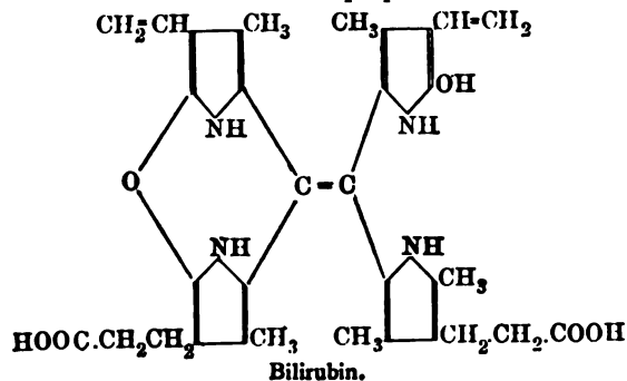
Bilirubin.
